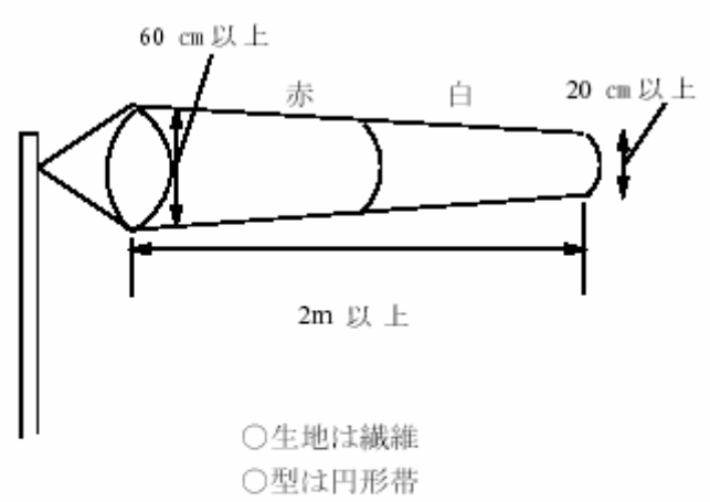
(b) 吹き流しの基準
