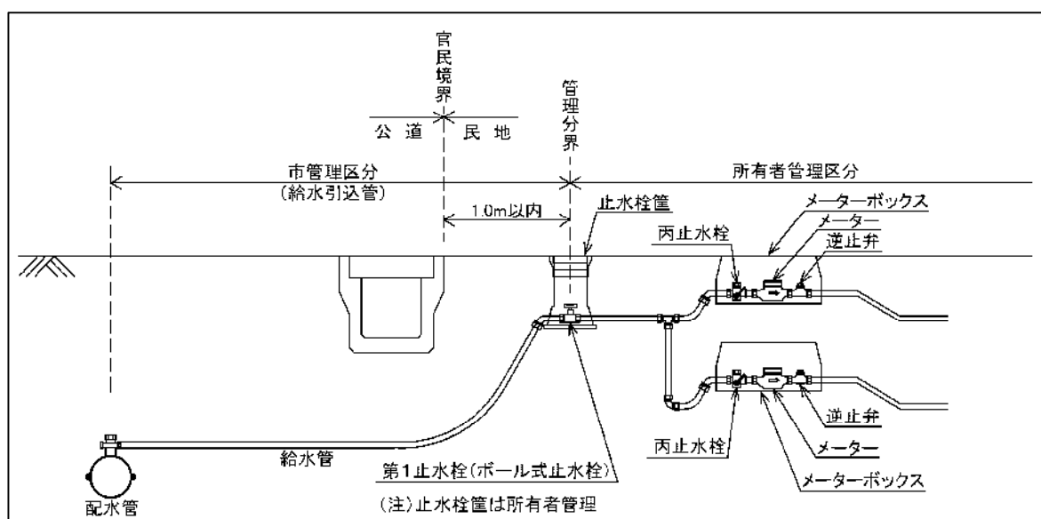
図 1 - 8 - 4 管理分界 (支管分岐の場合)
