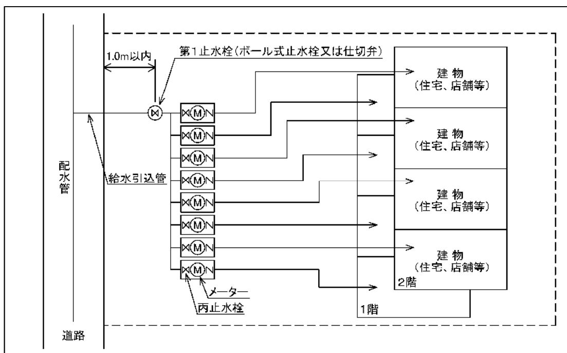
図 2 - 1 1 - 3 集合住宅（官民境界付近にメーターを設置）
